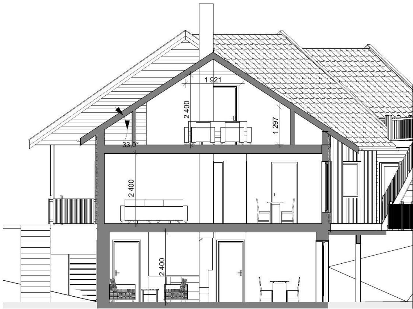
1:100 Snitt A
